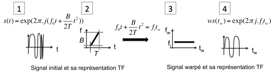
Figure 3. Représentation schématique de l'effet de déformation temporelle (warping temporel) sur une rampe de fréquences s(t) , avec t_w le temps déformé et f_i la fréquence de déformation, B la bande de fréquences et T la durée d'un écho
