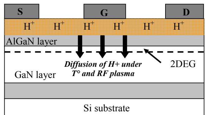
Fig. 1 Deuterium diffusion in AlGa N /Ga N structure
