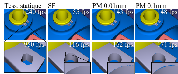
Figure 12: Examen de la qualité du rendu pour le modèle de piston. Tess. statique : tessellation statique de 0.1mm, SF : Schollmeyer et Fröhlich, PM : méthode proposée avec \epsilon = 0.01\text{mm} ou 0.1\text{mm} . Rendu effectué en tessellation dynamique avec une erreur d'écran de \epsilon_s = 0.1 . Temps de rendu fourni de manière indicative, exprimé en images par seconde (fps, de l'anglais frames per second).
