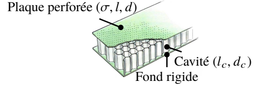
FIGURE 1 – Constitution d'un liner SDOF : superposition d'une plaque perforée et d'une cavité.
