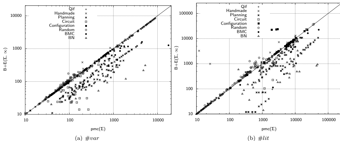
FIGURE 2 – Comparaison du nombre de variables et du nombre de littéraux de B + E(\Sigma) et de \text{pmc}(\Sigma) . Un point (x, y) correspond à une instance \Sigma pour laquelle la mesure vaut x pour \text{pmc}(\Sigma) et y pour B + E(\Sigma) .
