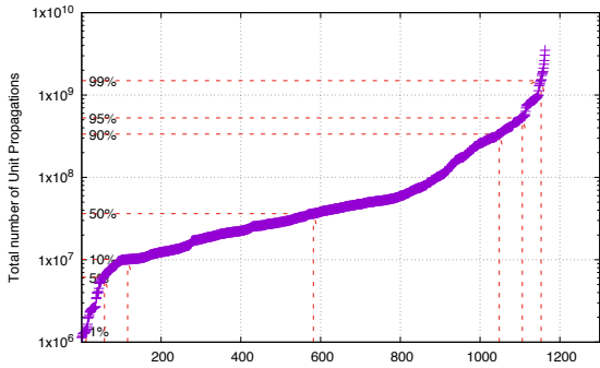
(a) Nombre de littéraux unitaires propagés
