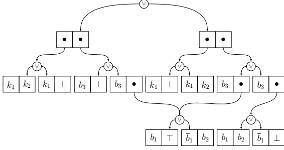
FIGURE 2 – Un circuit SDD_T représentant les contraintes d'un problème de configuration de maison.
