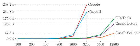
FIGURE 1 – Comparaison d'algorithmes de Time-Tabling : sur des instances de taille 100 à 12800, temps de descente sur une branche en utilisant une heuristique min-min.
