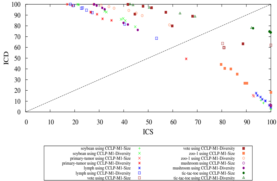
(a) CCLP-M1 : Diversité vs. taille de la description.
