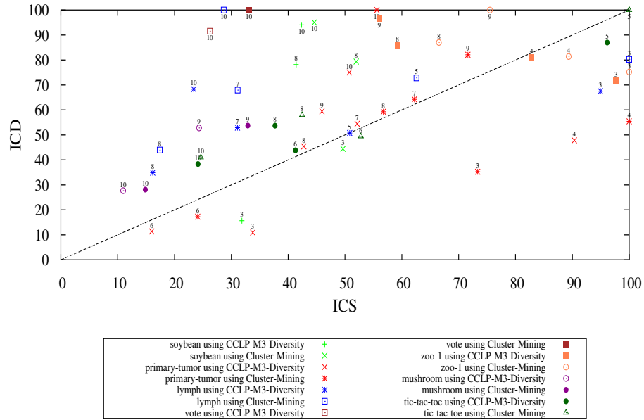
(a) CCLP-M3 avec la mesure de diversité vs. Cluster Mining (CM).
