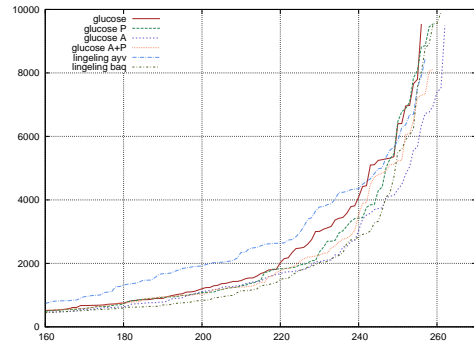
FIGURE 8 – Comparaison de différentes versions de Glucose et de lingeling sur les instances applications de la compétition SAT 2015. La table détaille le nombre d’instances SAT/UNSAT résolues, le graphique donne le cactus classique. Le temps est limité à 10000 secondes.
