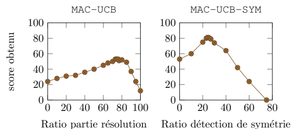
FIGURE 2 – Analyse de sensibilité pour MAC-UCB et MAC-UCB-SYM permettant de paramétrer l’exploitation, l’exploration et la détection de symétrie.
