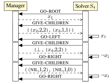
FIGURE 1 – Vue d’ensemble des messages échangés entre les solveurs S_4 et le MANAGER (Fig 1b) suivant une division de cubes sous forme d’arbre (Fig 1a) (une ligne pleine (resp. en pointillés) affecte la variable à vrai (resp. faux).
