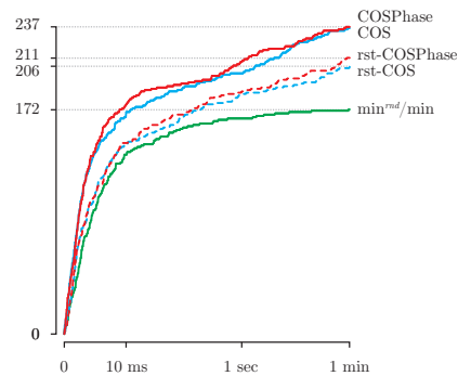
FIGURE 1 – Nombre d’instances résolues à l’optimal sous limite de temps. L’échelle des abscisses est logarithmique.
