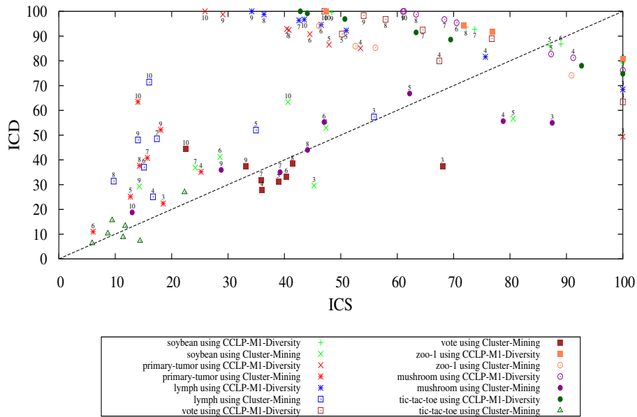
(b) CCLP-M1 avec la mesure de diversité vs. Cluster Mining (CM).
