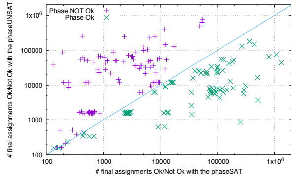
FIGURE 6 – Comparaison sur le nombre d’affectations qui sont en accord/désaccord entre le modèle et la phaseSAT ou la phaseUNSAT .
