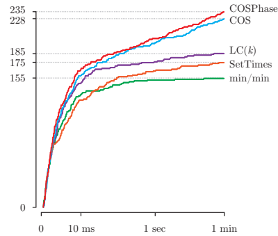
FIGURE 1 – Nombre d’instances résolues à l’optimal sous limite de temps. L’échelle des abscisses est logarithmique.
