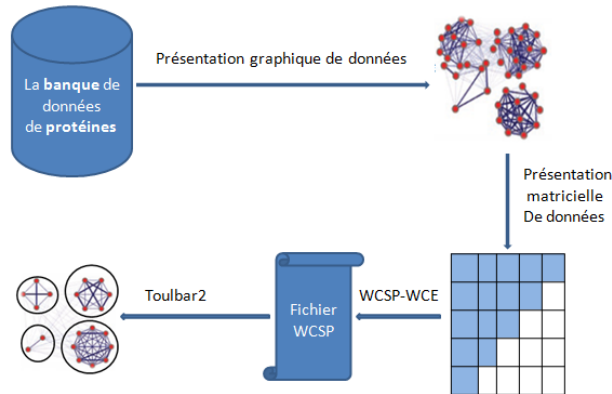
FIGURE 4 – Illustration des étapes de partitionnement de protéines en des cliques disjointes par le codage WCSP-WCE.
