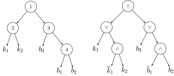
FIGURE 1 – Un vtrees T (gauche) et un circuit DNNF_T (droite).
