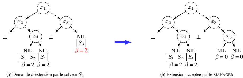
FIGURE 2 – La figure de gauche représente l’arbre avant l’extension. Comme la valeur de \beta satisfait le critère d’extension, le MANAGER l’accepte et modifie l’arbre pour obtenir celle de droite.
