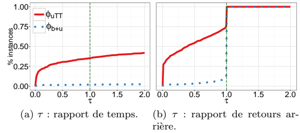
FIGURE 1 – Profils de performance pour les 960 instances.
