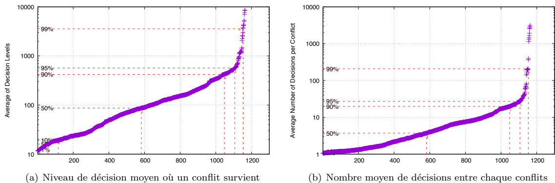
FIGURE 1 – Distribution cumulative auprès des 1162 problèmes. Statistiques collectées après 100000 conflits. Notez l'échelle logarithmique sur l'axe des ordonnées.
