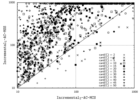
FIGURE 4 – Comparaison des temps de résolution (en secondes) entre Incremental 2 -AC-MCS et Incremental 1 -AC-MSS.
