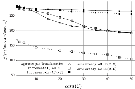
FIGURE 2 – Nombre d’instances résolues.
