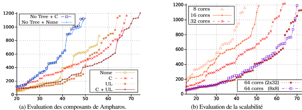
FIGURE 4 – Comparaison de plusieurs versions de AMPHAROS et évaluation de la scalabilité
