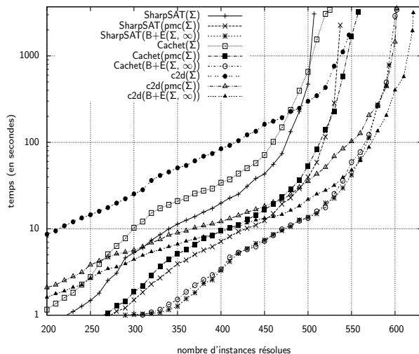
FIGURE 1 – Nombre d’instances résolues par Cachet, sharpSAT et C2D pour les prétraitements \emptyset , pmc et B + E. Un point (x, y) indique que le compilateur concerné a résolu x instances avec un temps limite inférieur ou égal à y secondes pour chacune d’entre elles.
