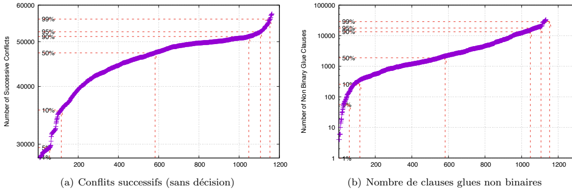
FIGURE 2 – Distribution cumulative auprès des 1162 problèmes. Statistiques collectées après 100000 conflits. Notez l'échelle logarithmique sur l'axe des ordonnées.
