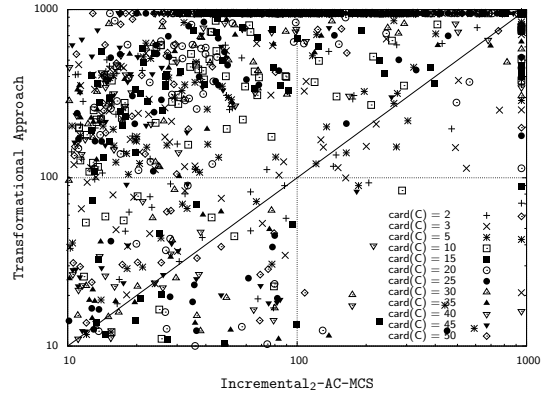
FIGURE 3 – Comparaison des temps de résolution (en secondes) entre Incremental 2 -AC-MCS et Approche de Transformation.
