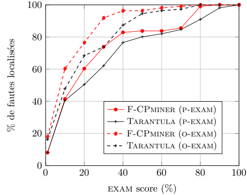
FIGURE 2 – TARANTULA et F-CPMINER : comparaison d'efficacité
