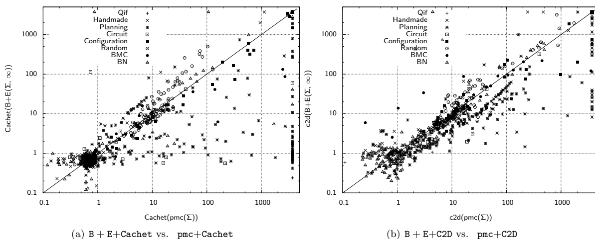
FIGURE 3 – Comparaison des performances en terme de temps de calcul pour déterminer le nombre de modèles des approches B + E + \text{Cachet} et \text{pmc} + \text{Cachet} , puis B + E + \text{C2D} et \text{pmc} + \text{C2D} . Un point (x, y) correspond à une instance \Sigma , pour laquelle le temps nécessaire au calcul du nombre de modèles est égal à x secondes quand \text{pmc} est le préprocesseur utilisé et y secondes quand il s’agit de B + E .
