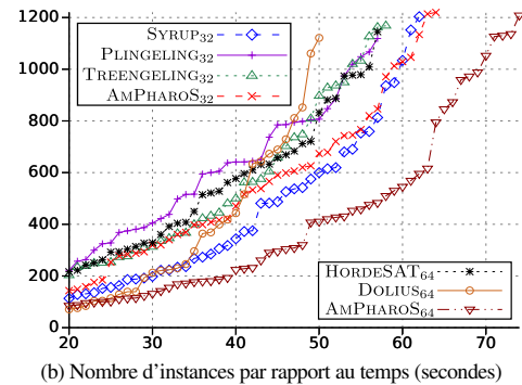
FIGURE 5 – Comparaisons d’AMPHAROS vs l’état de l’art des solveurs SAT parallèles. Le Tab. 5a donne les résultats de chaque solveur suivant le nombre de threads (#thr.).
