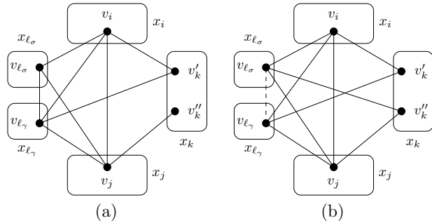
FIGURE 4 – Deux cas différents de deux valeurs v'_k et v''_k qui satisfont la 2-wBTP.
