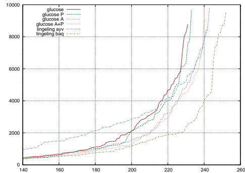
FIGURE 7 – Comparaison de différentes versions de Glucose et de lingeling sur les instances applications de la compétition SAT 2014. La table détaille le nombre d’instances SAT/UNSAT résolues, le graphique donne le cactus classique. Le temps est limité à 10000 secondes.
