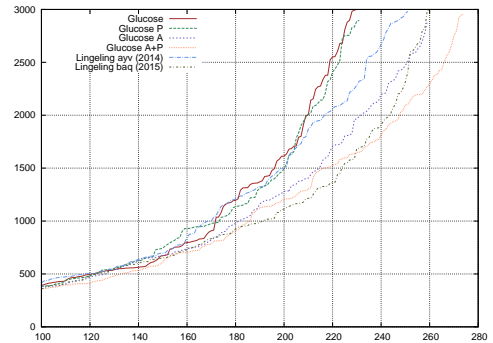
FIGURE 5 – Comparaison de différentes versions de Glucose et de lingeling sur un ensemble de 573 instances difficiles pour Glucose. La table détaille le nombre d’instances SAT/UNSAT résolues, le graphique donne le cactus classique. Le temps est limité à 3000 secondes.
