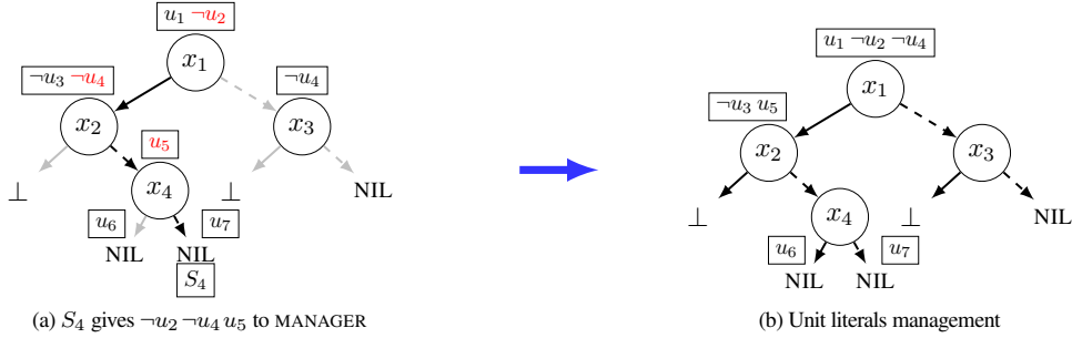
FIGURE 3 – La figure de gauche montre un arbre décoré avec les littéraux donnés par S_4 en rouge. Ces littéraux sont remontés, en utilisant deux règles (insatisfaisabilité pour u_5 et littéraux identiques pour \neg u_4 ) afin d’obtenir celle de droite.
