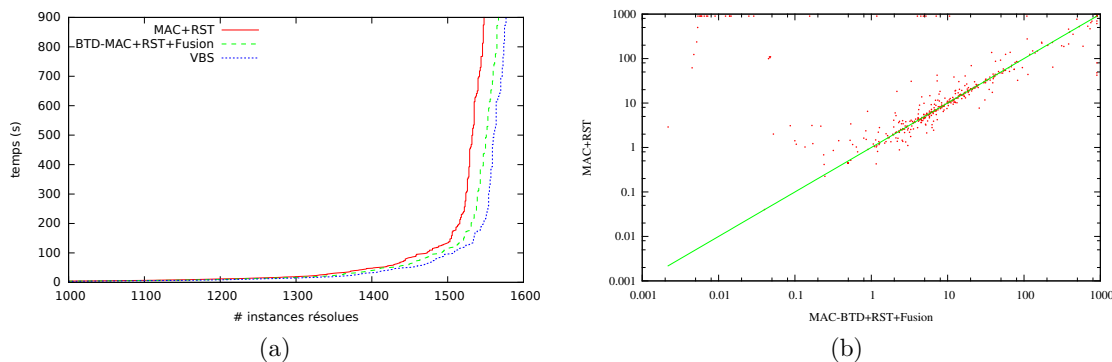
FIGURE 3 – (a) Nombre d’instances résolues pour MAC-BTD+RST+Fusion avec H_5 , MAC+RST et VBS, (b) comparaison des temps d’exécution de MAC-BTD+RST+Fusion et MAC+RST pour les 577 instances difficiles.
