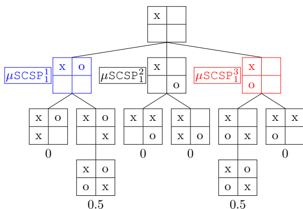
FIGURE 1 – L’arbre de recherche du Tic Tac Toe 2 × 2 avec les scores obtenus par MAC-UCB-SYM pour chaque état terminal
