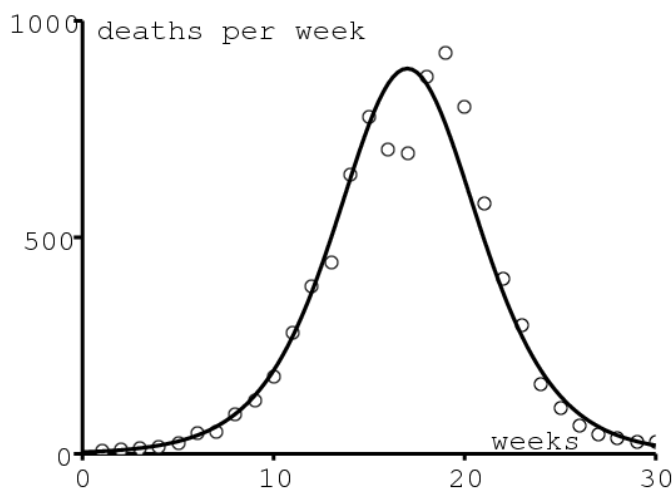
Рисунок 1. Число умерших от чумы в Бомбее за неделю с 17 декабря 1905 г. по 21 июля 1906 г. Advisory Committee, 1907b, p. 753). Уравнение кривой 890 / \cosh^2(0,2t - 3,4) как в (Kermack и McKendrick, 1927).
