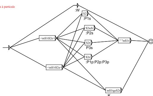
(a) Graphe de flexion pour les verbes à particule « met », « mit » ou « mit »
