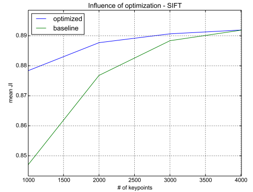
b) SIFT
