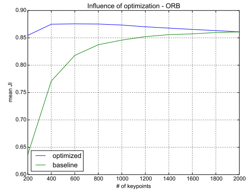
a) ORB
