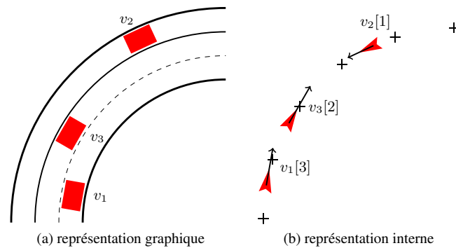
FIGURE 1. (a) Section de route avec un véhicule par voie. Représentation dans (b) TrafficGen : les carrefours sont des nœuds, chaque flèche est un vecteur de vitesse d'un agent véhicule, le nombre entre crochets indique le numéro de voie du véhicule
