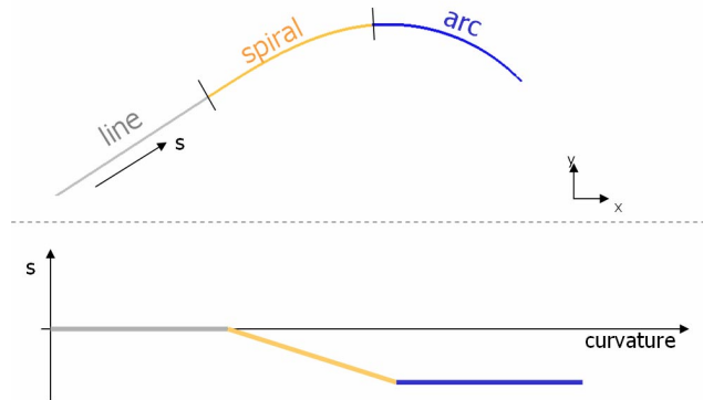
FIGURE 7. Extrait de la spécification OpenDrive illustrant les différentes géométries. La courbe du haut montre le rendu géométrique de chaque géométrie en fonction du coefficient de courbure (graphique du bas)
