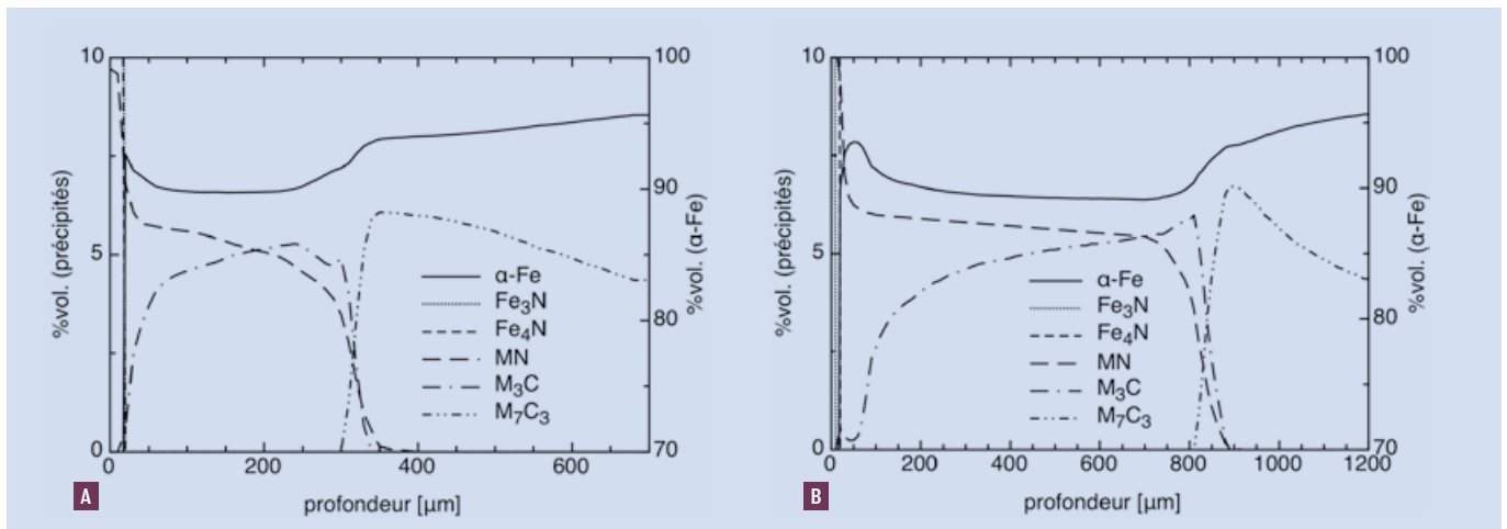
FIGURE 7 : Evolution de la fraction de phases à l'équilibre thermodynamique de l'acier Fe-3%Cr-0.35%Mn.C nitruré à 550 °C pendant (a) 10 et (b) 100 h. Les résultats sont calculés à partir de Thermo-Calc et des profils de composition chimique de la Figure 4.
