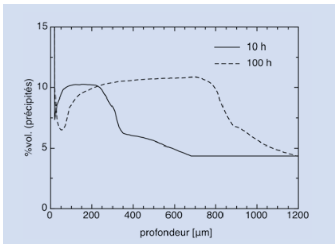
FIGURE 8A : Evolution de la fraction volumique totale de précipités de l'acier Fe-3%Cr-0.35%Mn.C nitruré à 550 °C pendant 10 et 100 h. Les résultats sont calculés à partir de Thermo-Calc.
