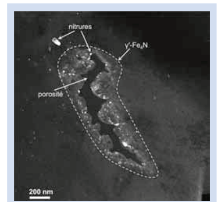
FIGURE 3 : Micrographie par microscopie électronique en transmission (en champ sombre) à 50 \mu\text{m} de profondeur de l'acier Fe-3% m.Cr-0.35% m.C nitruré à 550 °C pendant 100 h. Champ sombre à partir de l'intensité diffractée par les nitrures d'éléments d'alliage.
