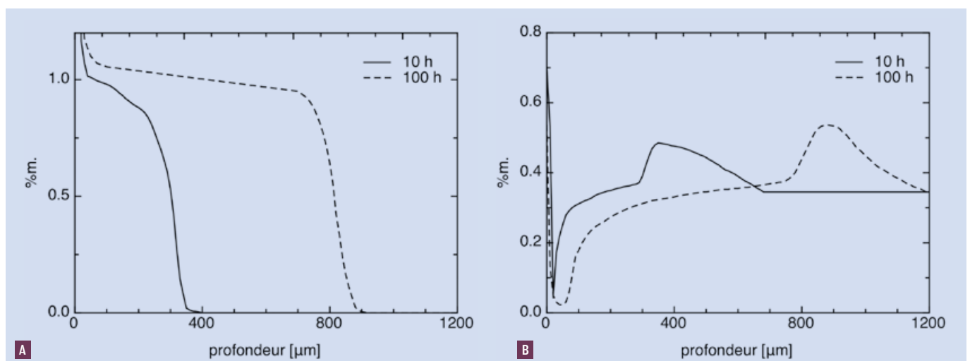
FIGURE 4 : Profils de composition chimique de l'acier Fe-3% m.Cr-0.35% m.C nitruré à 550 °C pendant 10 et 100 h. (a) azote (analyse par microsonde électronique à balayage) et (b) carbone (analyse par spectrométrie à décharge électroluminescente).
