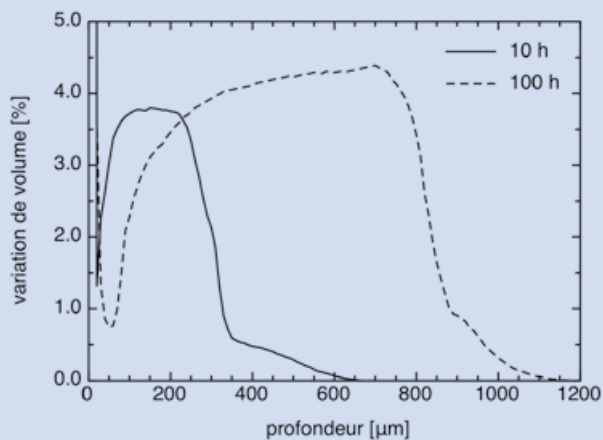
FIGURE 10 : Variations de volume calculées accompagnant la précipitation de l'acier Fe-3%Cr-0.35%Mn.C nituré à 550 °C pendant 10 et 100 h. La transformation des carbures n'est pas prise en compte.
