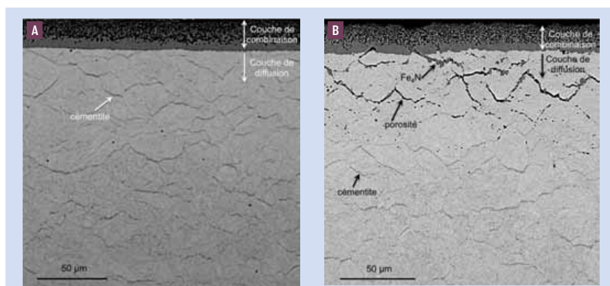
FIGURE 2 : Micrographies par microscopie électronique à balayage (image en électrons rétrodiffusés) de l'acier Fe-3% m .Cr-0.35% m .C nitruré à 550 °C pendant (a) 10 et (b) 100 h. Aucune attaque chimique préalable.
