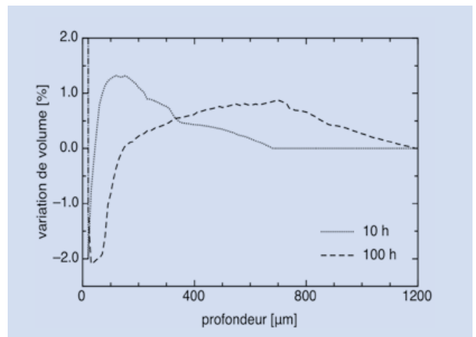
FIGURE 8B : Variations de volume calculées accompagnant la précipitation de l'acier Fe-3%Cr-0.35%Mn.C nitruré à 550 °C pendant 10 et 100 h. La composition du matériau à cœur est prise comme référence.
