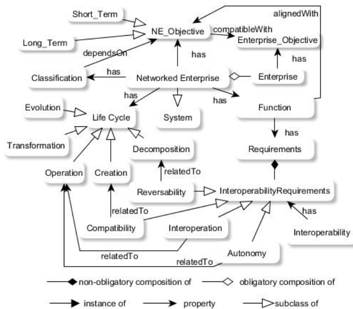
Fig. 2. The NEMO meta-model.
