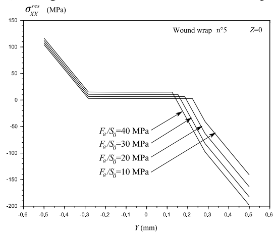
(d) Residual stress along thickness
