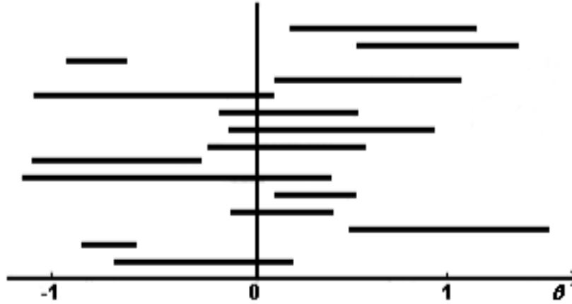
FIGURE 1 – Intervalles de confiance à 50%
