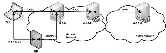
Fig. 4 PANA Framework
