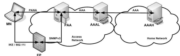
Fig. 4 PANA Framework
