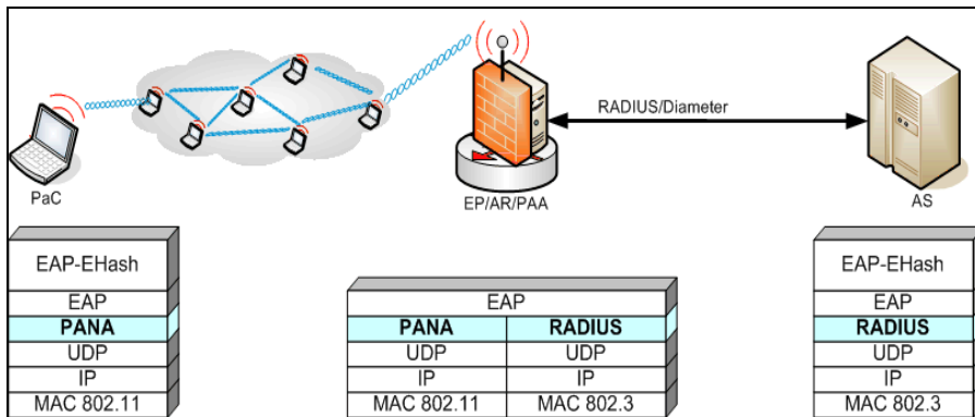
Figure 3. Encapsulation des paquets EAP pendant l'authentification PANA (EP/AR et PAA sont colocalisés)
