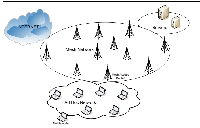
Figure 1. Architecture de réseau mesh multi sauts
