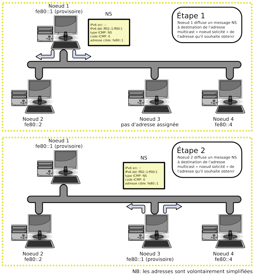
Fig. 1: La machine 1 et la machine 3 souhaitent une adresse qui n'est pas attribuée, mais qui est la même et ne pourront pas l'obtenir.
