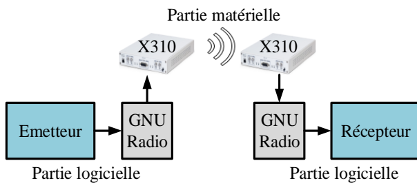
Figure 3. Sondeur de canal basé radio logicielle
