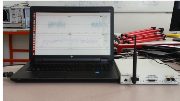
Figure 4. Banc de mesures
