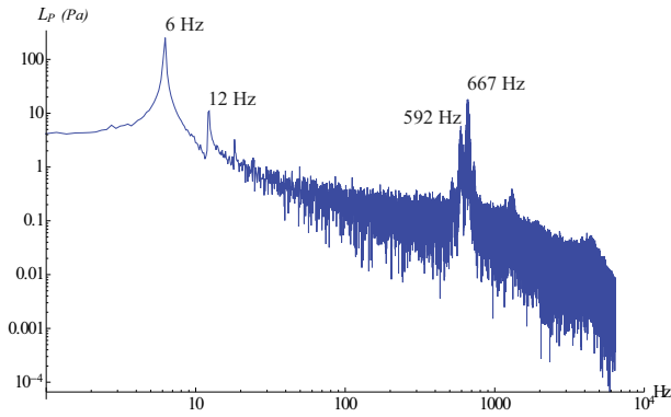
FIGURE 7 – Spectre de pression mesurée à 5 cm de l'extrémité aval du tuyau pour U = 20 m/s. Signal infrasonore à 6 Hz.
