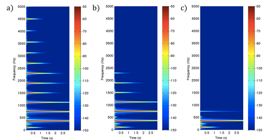
Figure 9 – Spectrogramme de la pression rayonnée à 1,5m en face de la table pour différentes excitations. a) Porte ; b) Fortissimo ; c) Pianissimo.
