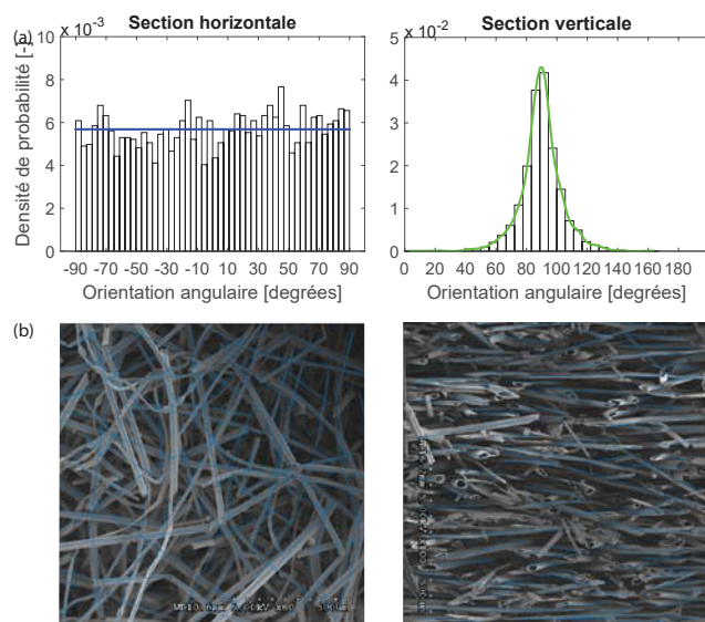
Figure 1: (a) Distributions de l'orientation des fibres déterminées expérimentalement par Microscopie Electronique à Balayage (MEB). Les histogrammes sont convertis en densités de probabilités. (b) Images MEB correspondant à des sections horizontale (plan xy ) et verticale (plan orthogonal à xy ).
