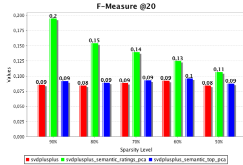
FIG. 1 – Métrique "F-mesure".
