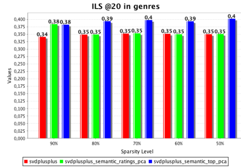
FIG. 2 – ILS in "genre" attribute.
