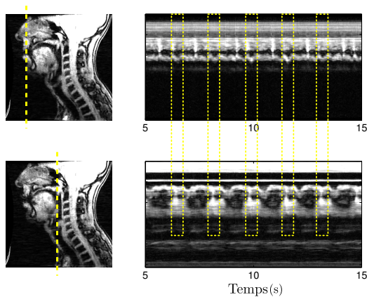
FIGURE 3 – Tracés en bande de répétitions de la phrase "J'ai pigé la phrase" (/ʒe.pi.ʒe.la.fʁɑz/). Haut : tracé en bande au niveau des lèvres. Bas : tracé en bande de la constriction uvulaire. Les positions des coupes sont indiquées par la ligne verticale sur les coupes médio-sagittales à gauche. Les boites sur les tracés de droite indiquent les moments de la production du mot "phrase" (/fʁɑz/). La résolution temporelle est de 35 ms. La résolution spatiale est de 1.016 \times 1.016 \text{ mm}^2 , et l'épaisseur de coupe est de 5 mm.
