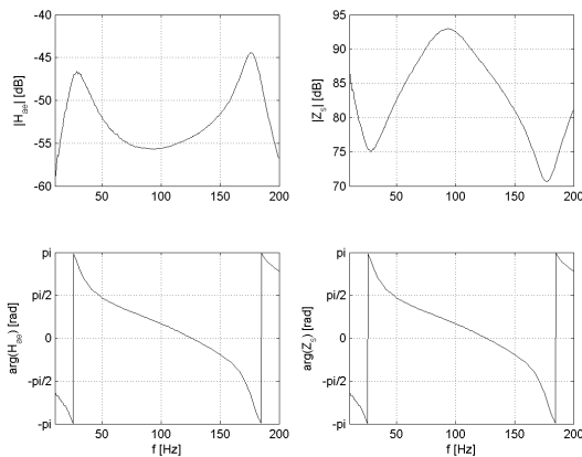
FIGURE 4 – H_{ae} et Z_s estimées au microphone M_1 .
