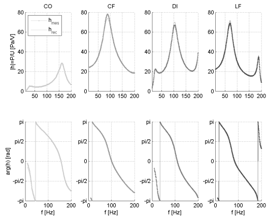
FIGURE 5 – Comparaison de h_{mes}^1 (ligne pointillée) et h_{rec}^1 (ligne continue) pour les 4 terminaisons au microphone M_1 .
