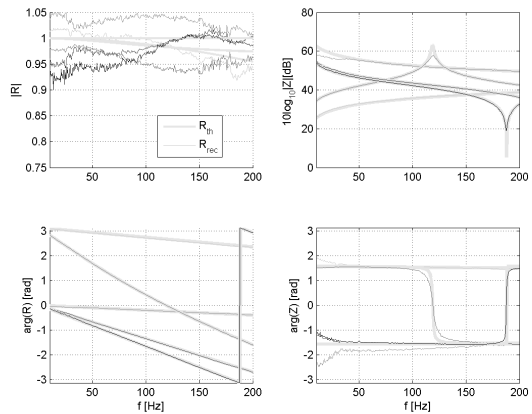
FIGURE 6 – Comparaison des impédances et coefficient de réflexion théorique et reconstruit pour les 4 terminaisons au microphone M_1 .
