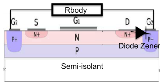
Fig. 2. Schéma du planar MESFET avec Zener sur l'électrode de drain.
