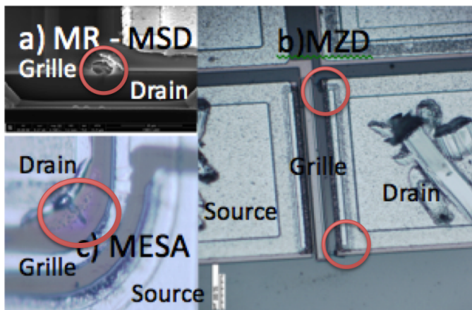
Fig. 4. Localisation de défaut après stress TLP sur différents MESFET (a) MR-MSD (b) MZD (c) Mesa MESFET.
