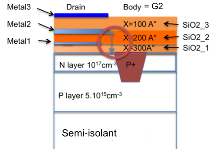
Fig. 12. Schéma de la structure de MR avec ses épaisseurs d'oxyde de passivation.
