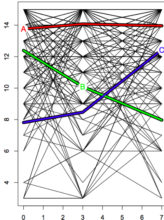
Figure 2 Représentation d'une modélisation en K-means longitudinaux en 3 groupes sur les données réelles (N = 234)
