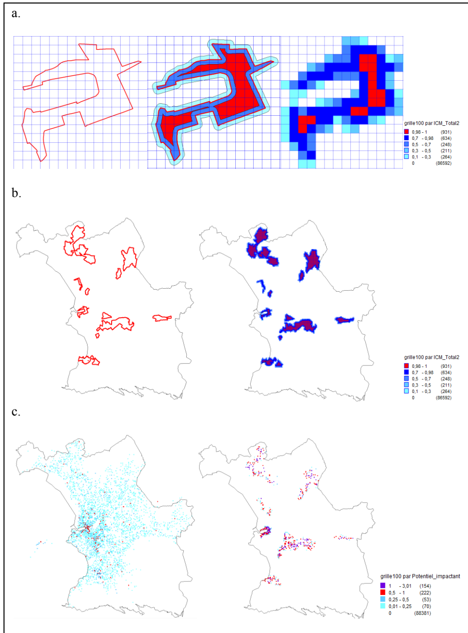
Figure 1. a. Exemple de fuzzyfication d'un périmètre de zone inondable (secteur du périmètre de zone inondable (secteur du vieux port) b. Méthodes appliquées aux zones (Iris) de la commune de Marseille citées au moins une fois dans la presse comme zones inondées entre 1951 et 2003 (pour 5 évènements de référence, 1951, 1978, 1993, 2000 et 2003) c. Estimation de la susceptibilité par croisement aux nombres de postes électriques
