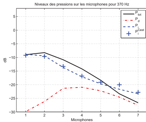
FIGURE 9 – Comparaison des pressions incidentes exactes P_i et estimées contrôlées P_i^{Cest} pour une source à 370Hz
