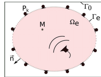
FIGURE 3 – Schéma de principe d'estimation du champ diffracté des parois
