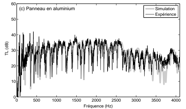
FIGURE 6 – Comparaison des résultats de simulation et expérimentaux pour les deux panneaux : (a) Fréquences propres théoriques et expérimentales - (b,c) TL en bandes fines pour les deux panneaux considérés (simulation : calcul éléments finis).
