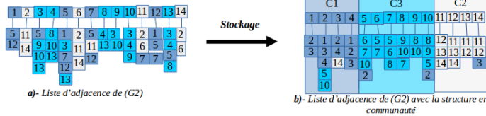
Figure 4 – Liste d’adjacence de (G2) tenant compte des communautés
