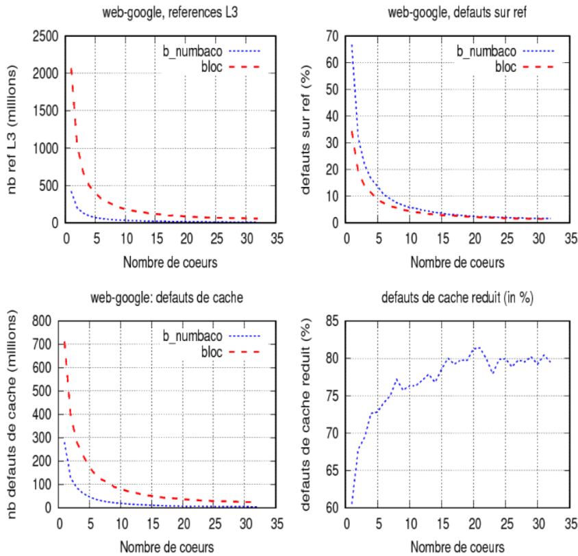
Figure 12 – Réduction des défauts de cache – web-google, Pagerank
