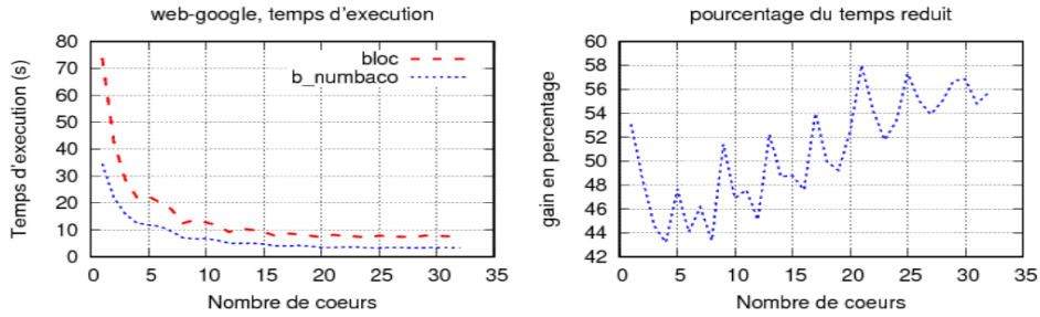
Figure 11 – Réduction du temps d’exécution – web-google, Pagerank La différence de performance entre le Pagerank (80% des défauts de cache pour 50% du temps d’exécution) et le score de Katz (73% des défauts de cache pour 21% du temps d’exécution) s’explique l’exploration locale (Propriété 3.1) : dans le cas du Pagerank, les
