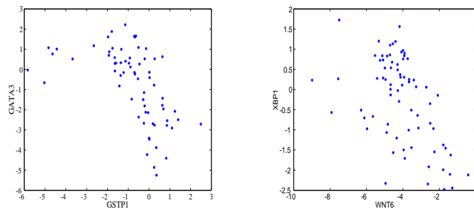
FIG. 3: Comparaison de gènes anti-corrélés : GATA3–GSTP1 (à gauche) et WNT6–XBP1 (à droite).
