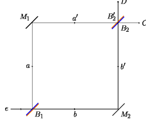
Fig. 3. Mach-Zehnder interferometer
