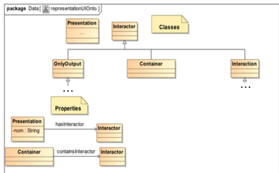
Figure 1. UIOnto
