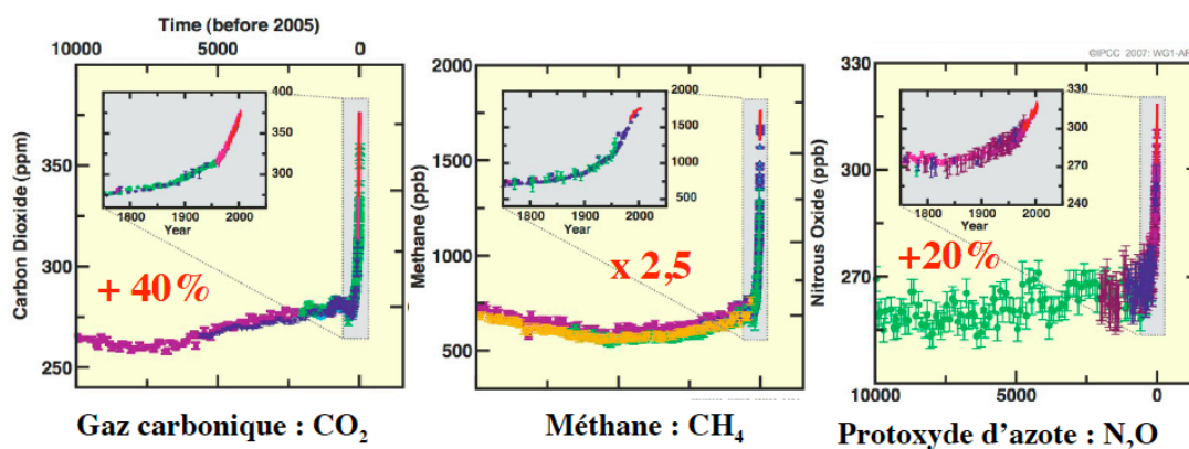
Evolution des principaux gaz à effet de serre
