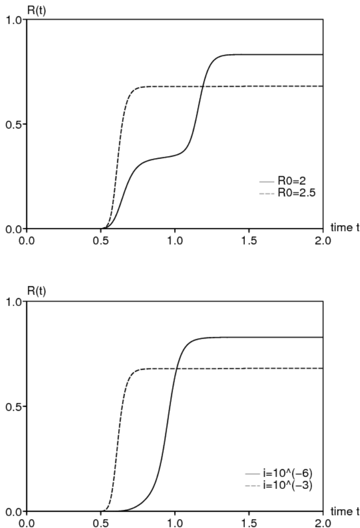
图1.该流行病的最终规模可能不会增长: a) 具有可复制性 \mathcal{R}_0 ; b) 初始分数 i 的感染者。
