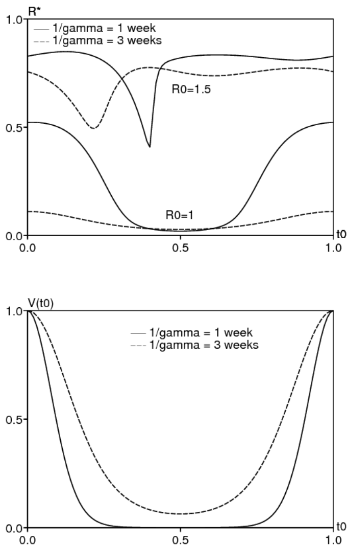
图3. (a) 如果 \mathcal{R}_0 接近1, 疫情的最终规模很大程度上取决于 t_0 如果传染期比季节长短。 (b) 标准化的“生殖价值” V(t_0) 给出了流行病最终规模对 t_0 (这里, \mathcal{R}_0 = 1 ) 。
