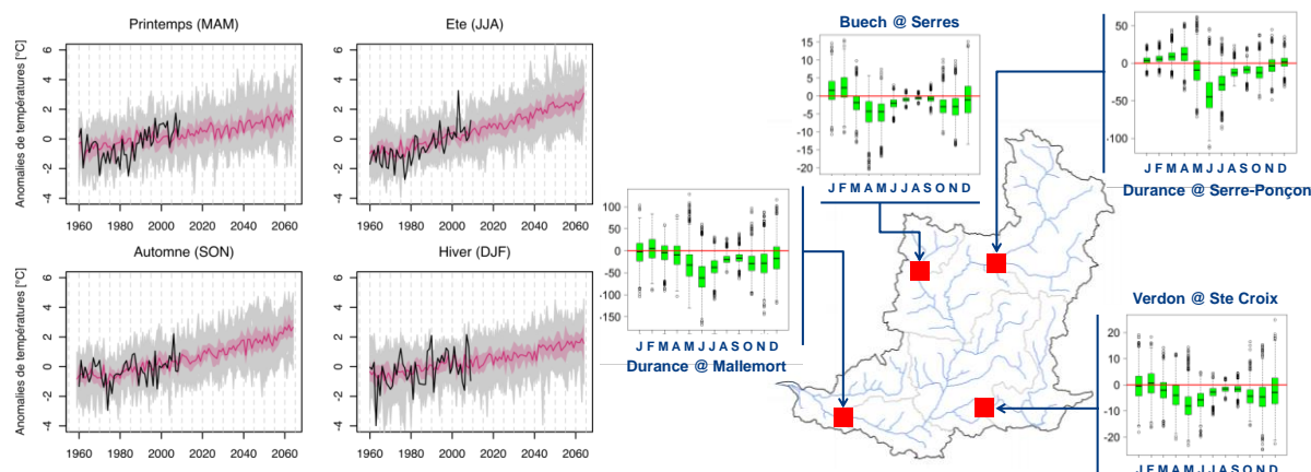
Figure 3 : Evolution des anomalies de températures saisonnières moyennes du bassin de la Durance à sa confluence avec le Rhône et de débits mensuels exprimés en m 3 /s sur la période 2036-2065 (à gauche : les anomalies des 330 projections climatiques sont tracées en gris, la médiane est en rose foncé et l'enveloppe rose est l'intervalle entre les premier et troisième quartiles ; les forçages DuO sont représentés en noir ; à droite : les boîtes à moustache sont définies par l'intervalle inter-quartile par rapport à la période de référence 1980-2009
