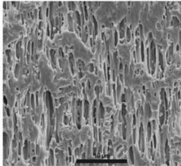
c) \epsilon_{33} = 1.4
