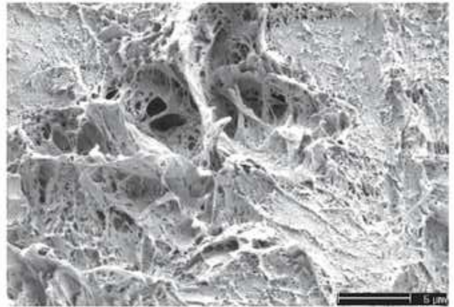
b) \epsilon_{33} = 0.48
