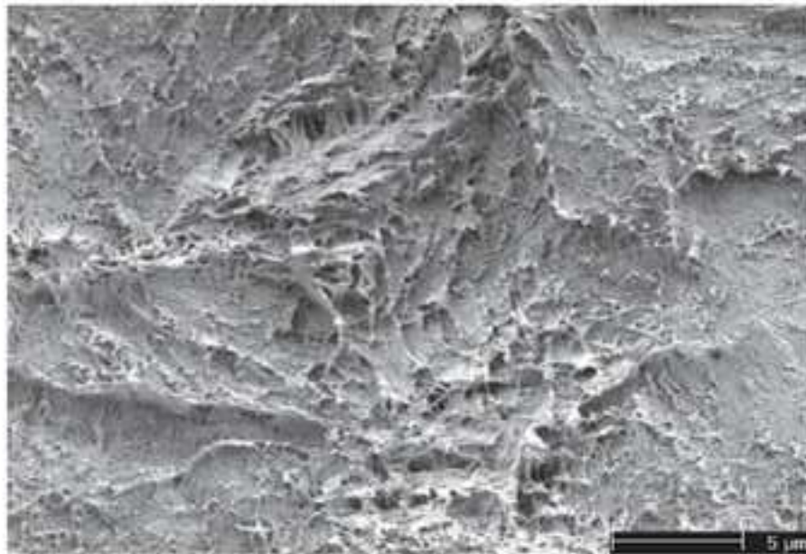
a) \epsilon_{33} = 0.29
