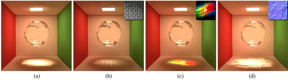
Figure 4: Utilisation de textures pour contrôler l'édition (a) La scène d'origine. (b) Utilisation d'une texture pour contrôler \lambda . (c) Utilisation d'une texture pour contrôler \theta . (d) Utilisation d'une carte de normales pour contrôler M_d .
