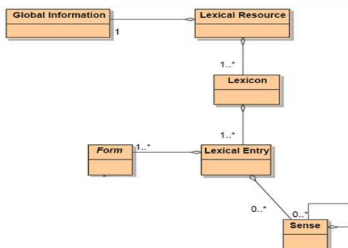
Figure 3 Noyau du méta-modèle LMF
