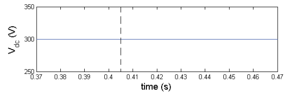
Fig. 22. DC-link voltage- case 3.
