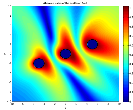
(d) Absolute value of the scattered field
