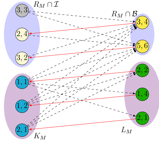
FIG. 2 – Ensembles de réduction
