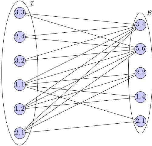
FIG. 1 – Graphe de compatibilité pour un problème de Vector Packing
