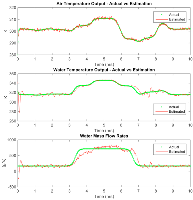
Fig. 4. State and parameter estimates: q_w estimation
