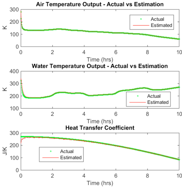
Fig. 2. State and parameter estimates: U_A estimation
