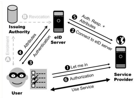
Fig. 6. Mediation with user control (D)
