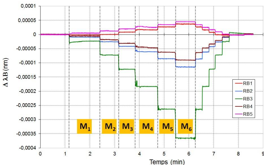
Figure 5 : Evolution de la longueur de Bragg des 5 RB en fonction des 6 cas de chargement
