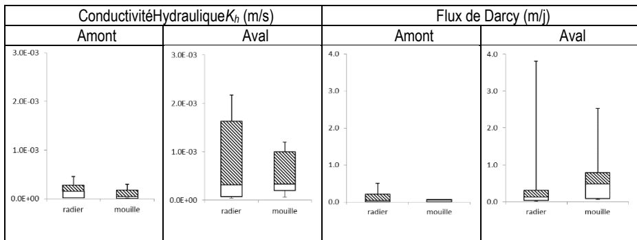
Figure 4 : Distributions des flux de Darcy et de K des radiers et des mouilles des deux tronçons.
