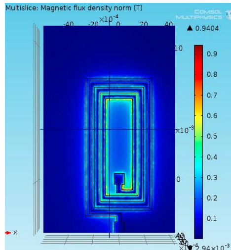
Figure 1 : Distribution de densité du flux magnétique le long de la micro-bobine
