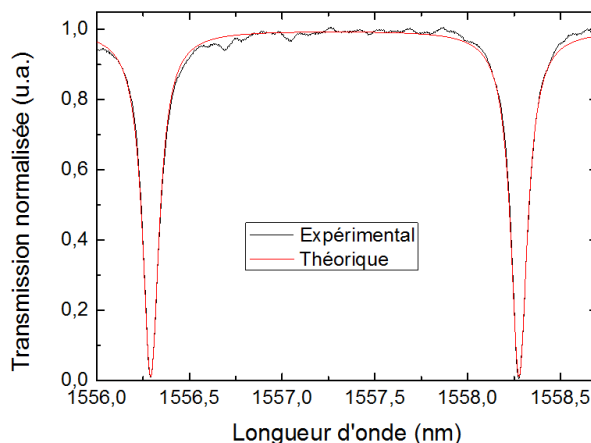
Fig. 3: Spectres de transmission expérimental et théorique, obtenus pour un micro-résonateur de gap 0,5 \mu\text{m} avec de l'eau en superstrat.
