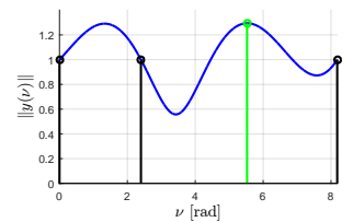
Fig. 10. Primer vector norm: First iteration.
