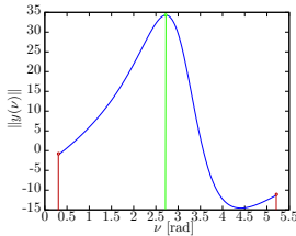
Fig. 4. Primer vector norm: Initialization.
