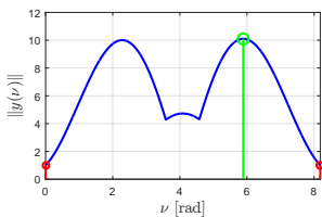
Fig. 13. Primer vector norm: Initialization.
