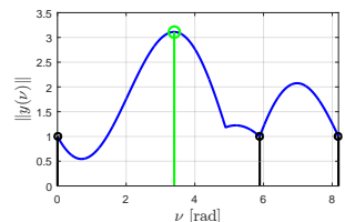
Fig. 14. Primer vector norm: First iteration.
