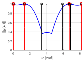
Fig. 15. Primer vector norm: Final iteration.
