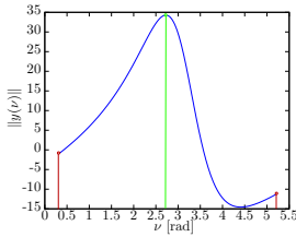
Fig. 4. Primer vector norm: Initialization.
