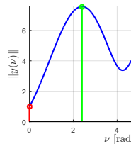
Fig. 9. Primer vector norm: Initialization.
