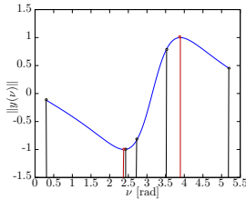
Fig. 6. Primer vector norm: Final iteration.
