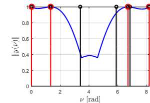
Fig. 15. Primer vector norm: Final iteration.
