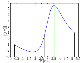
Fig. 5. Primer vector norm: First iteration.
